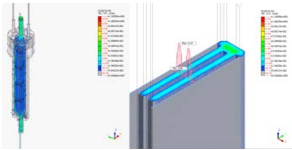
살균수 생성효율에 미치는 유속, 살균수 체류 시간에 대한 유동해석
