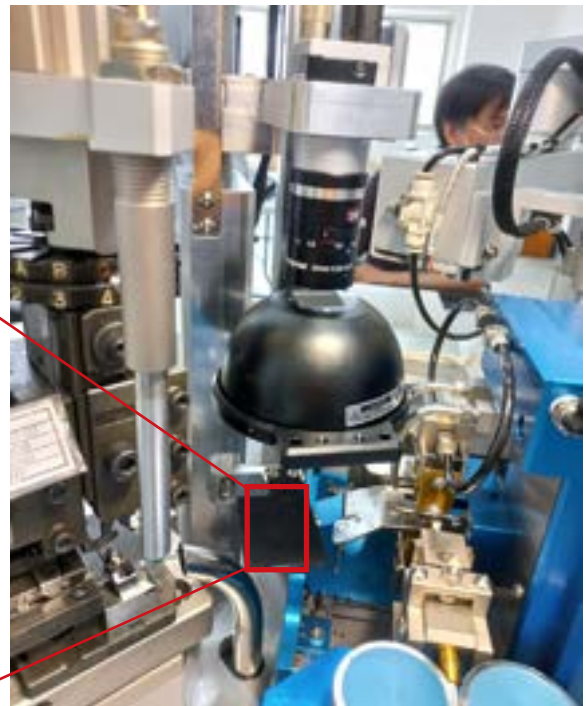
실시간 압착 검사 시스템 (CVM)
