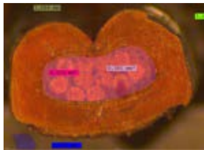
압착 단자 단면
